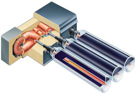
Abb.3: Vakuumröhrenkollektor
