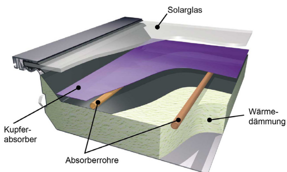
Abb.2: Aufbau eines Flachkollektors
