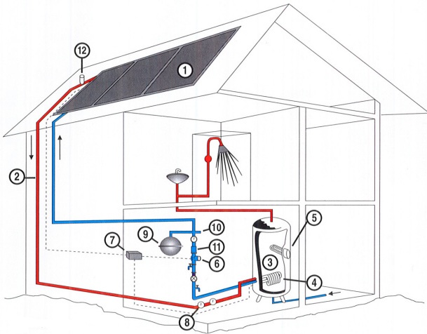
Abb. 1: Solaranlage schematisch
